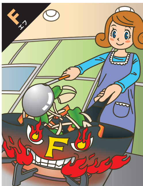
原子番号 9 フッ素(ふっそ) 元素記号 F
