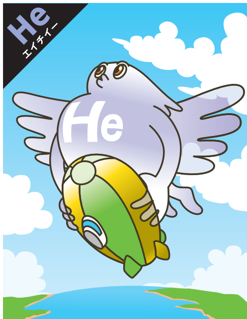
原子番号 2 ヘリウム 元素記号 He
