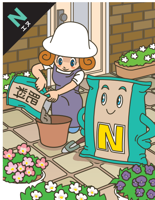
原子番号 7 窒素(ちっそ) 元素記号 N
