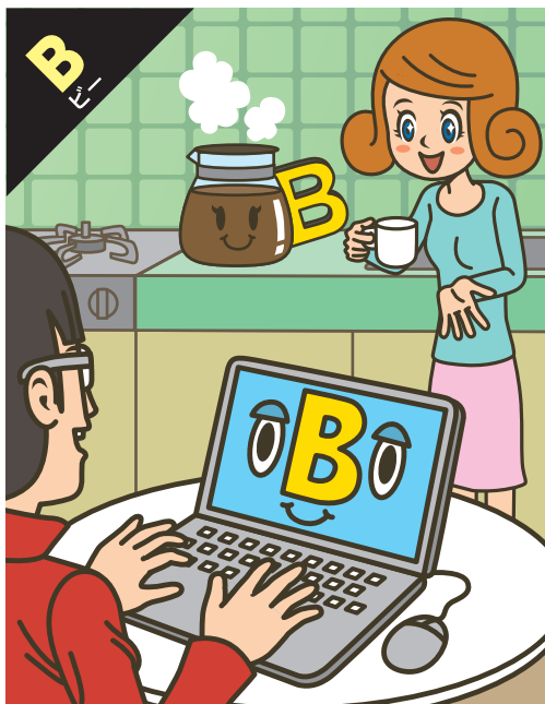
原子番号 5 ホウ素(ほうそ) 元素記号 B
