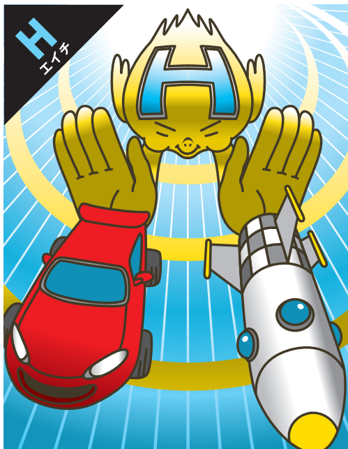
原子番号 1 水素(すいそ) 元素記号 H
